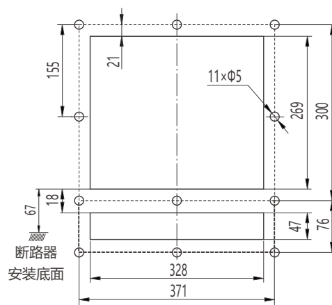
RDW7-4000~6300抽屉式断路器面板开孔尺寸
