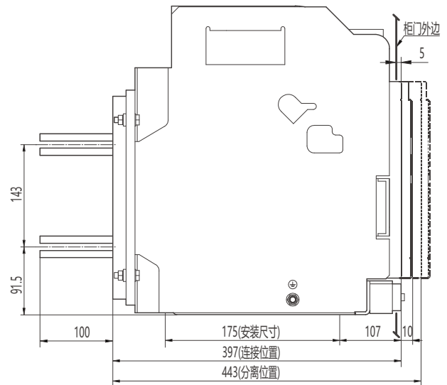
水平接线及外形尺寸
