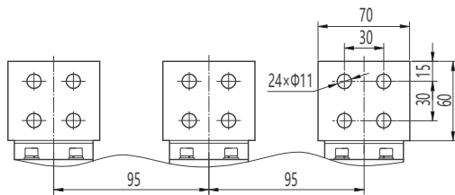
水平接线及相间距
