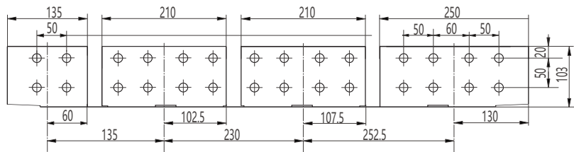
四极水平接线及相间距
