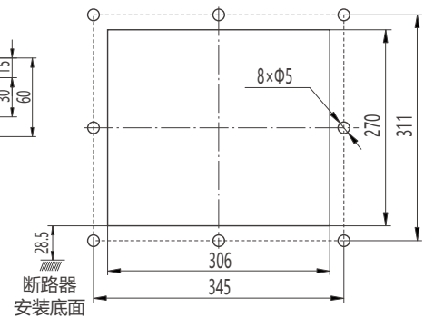
RDW7-2500固定式断路器面板开孔尺寸
