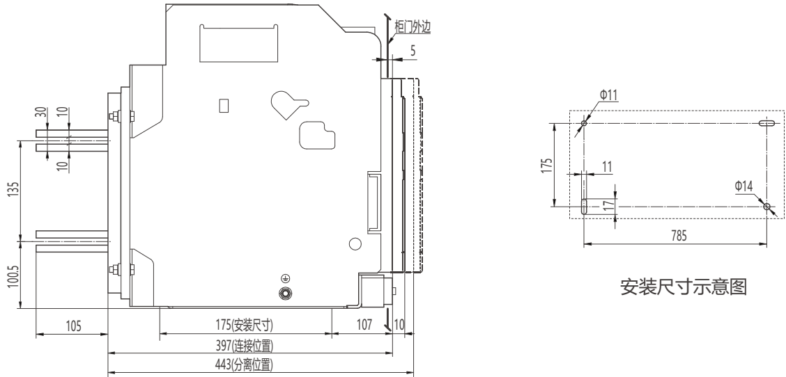
水平接线及外形尺寸
