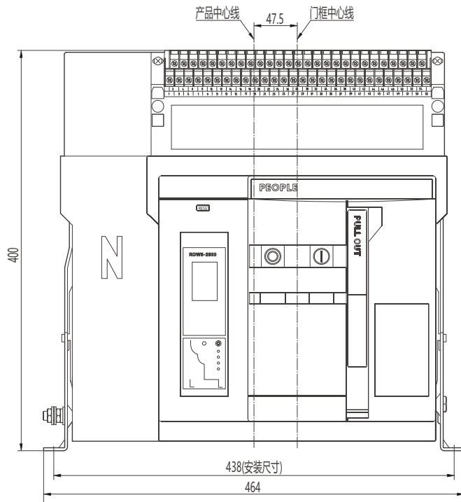
中心线及外形尺寸
