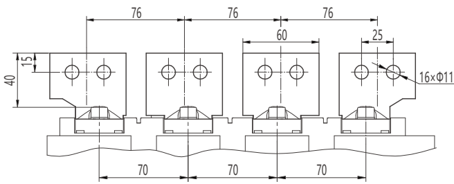
水平接线及相间距
