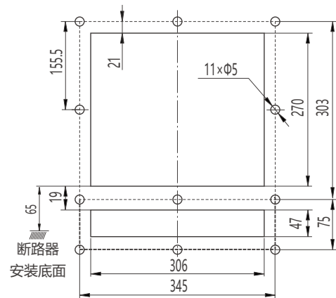
RDW7-2500抽屉式断路器面板开孔尺寸
