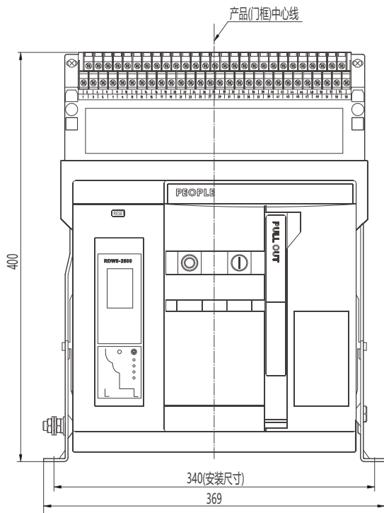
中心线及外形尺寸
