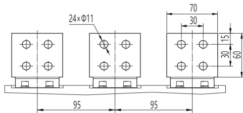
水平接线及相间距
