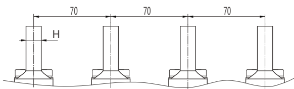
垂直接线及相间距
