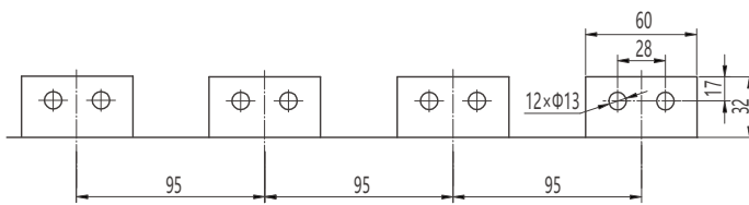
水平接线及相间距
