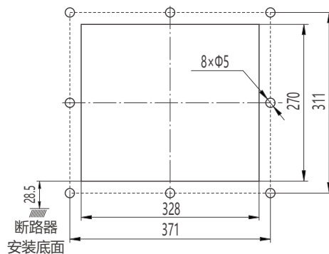
RDW7-4000 ~ 6300固定式断路器面板开孔尺寸
