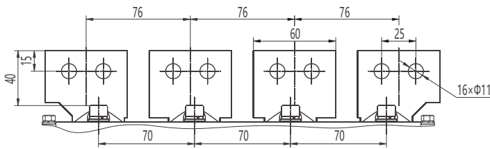
水平接线及相间距
