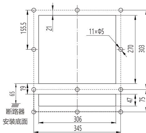
RDW7-2500S抽屉式断路器面板开孔尺寸
