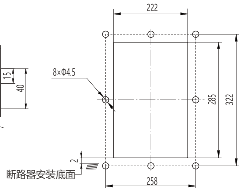
RDW7-1600固定式断路器面板开孔尺寸
