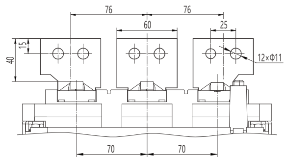
水平接线及相间距
