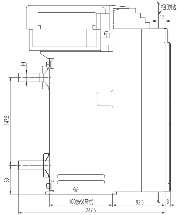
水平接线及外形尺寸
