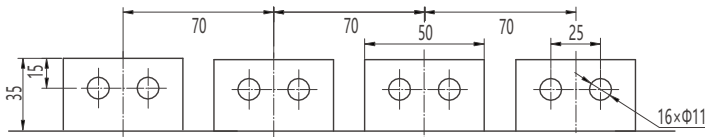
水平接线及相间距
