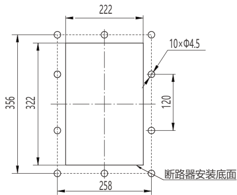
RDW7-1600S抽屉式断路器面板开孔尺寸
