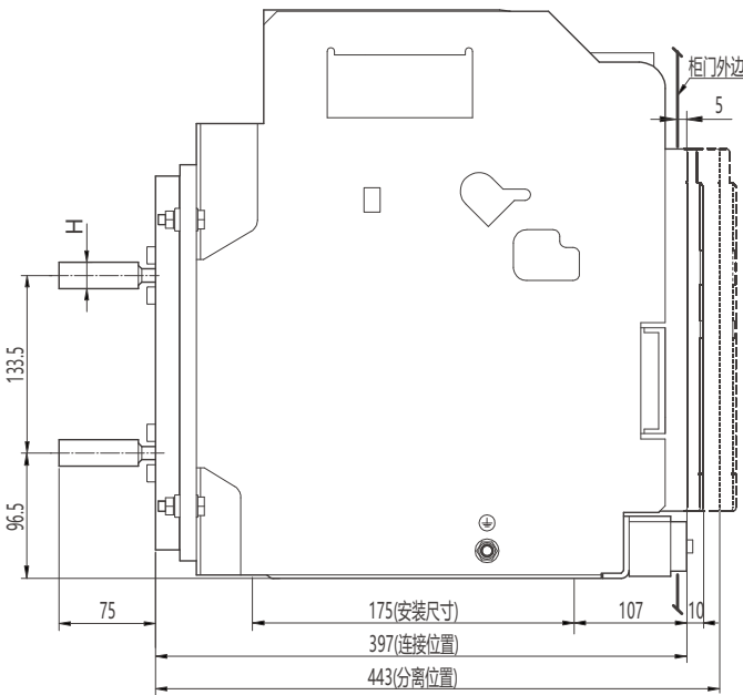
水平接线及外形尺寸
