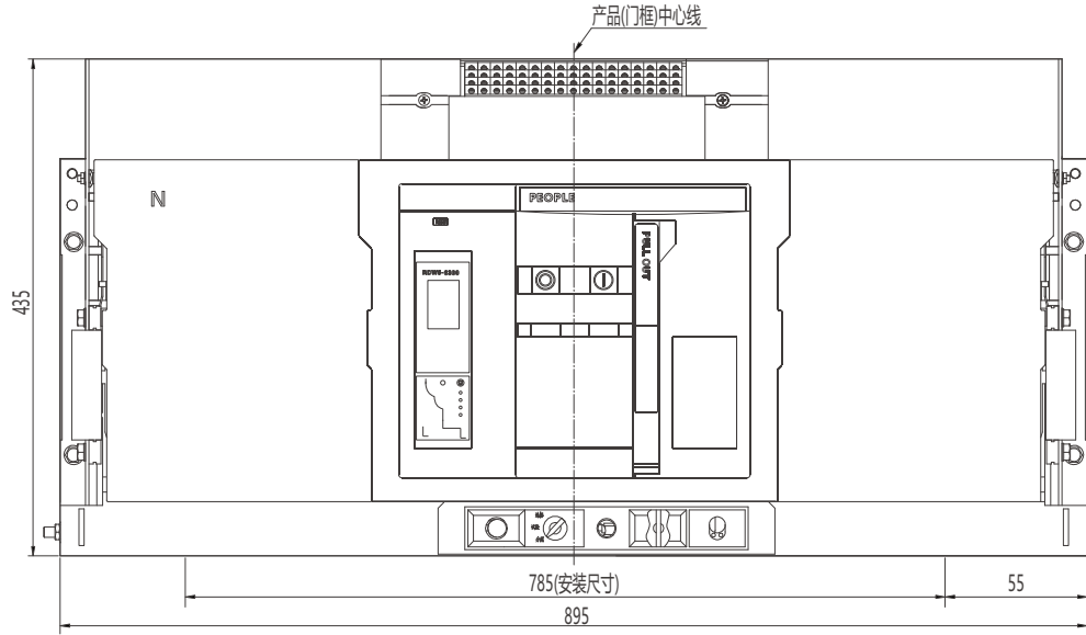
中心线及外形尺寸
