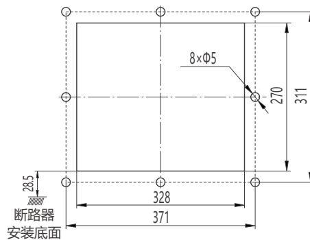
RDW7-4000 ~ 6300固定式断路器面板开孔尺寸
