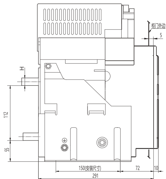
水平接线及外形尺寸
