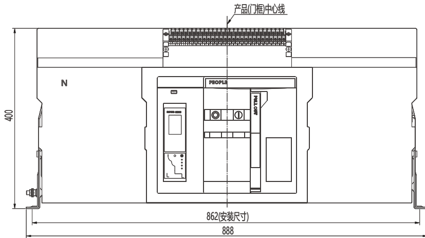
中心线及外形尺寸
