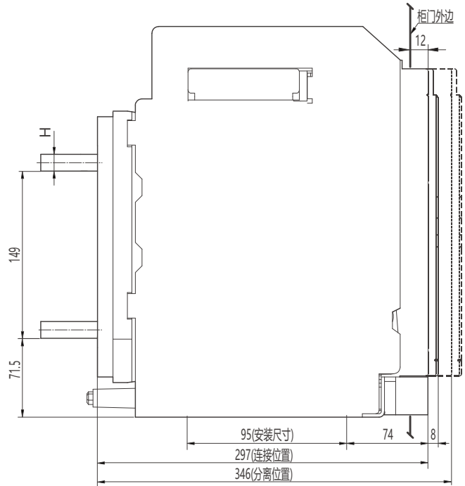
水平接线及外形尺寸
