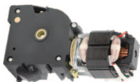
RDW7-1600(S)储能电机
