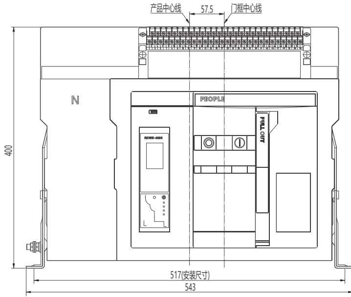
中心线及外形尺寸
