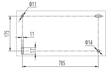
安装尺寸示意图
