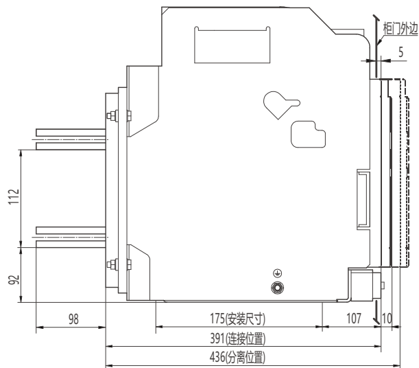
水平接线及外形尺寸
