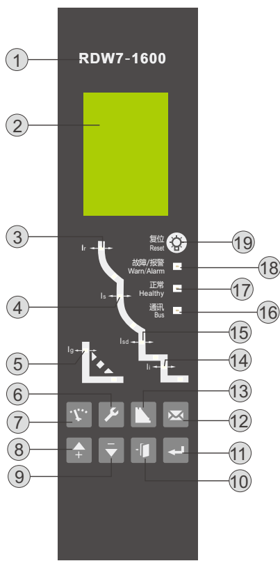
RDW7-1600智能控制器界面
