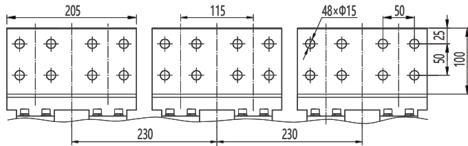
水平接线及相间距
