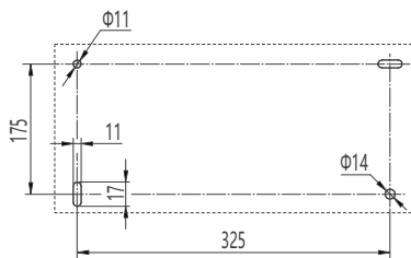
安装尺寸示意图
