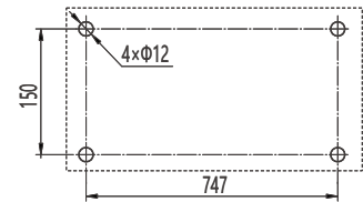
安装尺寸示意图
