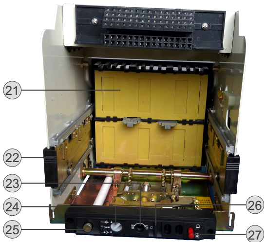
抽屉座
