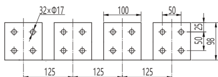
水平接线及相间距
