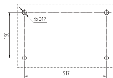
安装尺寸示意图
