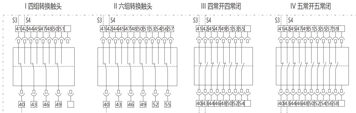
RDW7-2500 ~ 6300M型二次回路接线图
