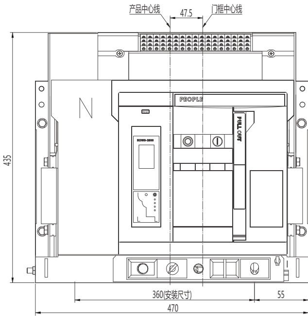
中心线及外形尺寸
