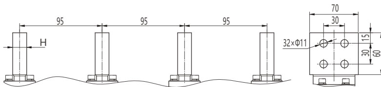
垂直接线及相间距
