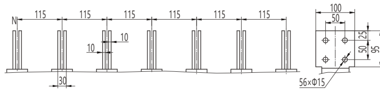
垂直接线及相间距
