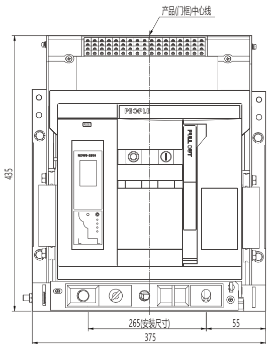
中心线及外形尺寸
