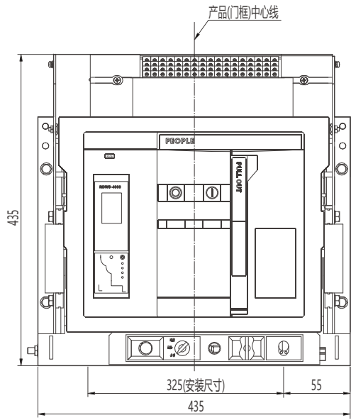
中心线及外形尺寸
