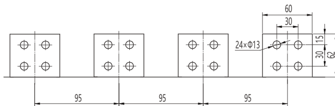
特殊订货水平接线及相间距
