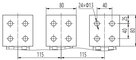
水平接线及相间距
