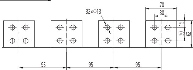
水平接线及相间距
