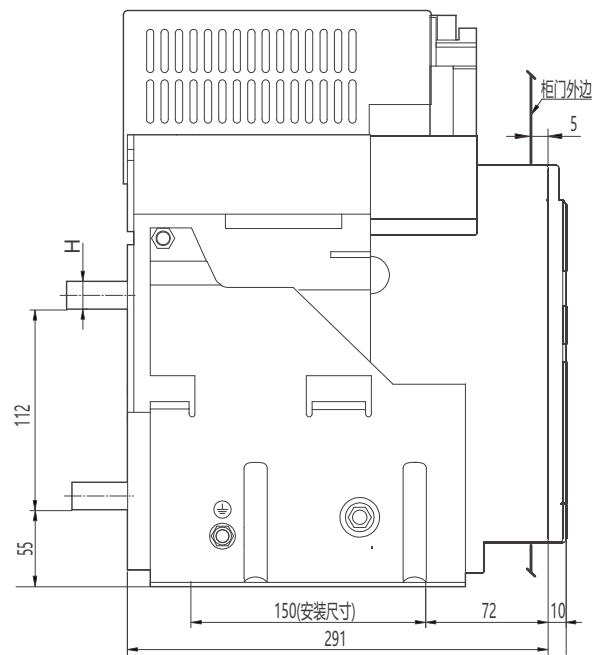
水平接线及外形尺寸
