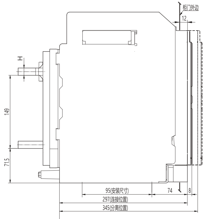
水平接线及外形尺寸
