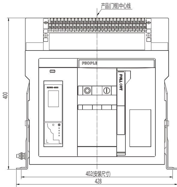
中心线及外形尺寸
