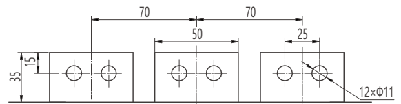
水平接线及相间距
