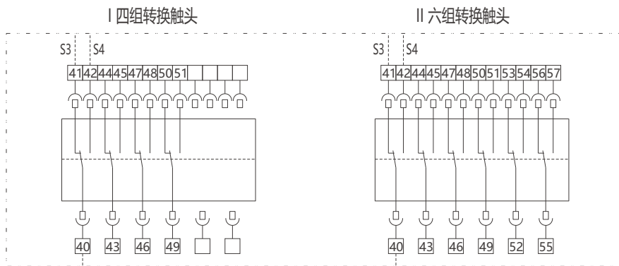
RDW7-1600M型二次回路接线图
