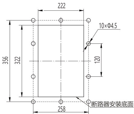
RDW7-1600S抽屉式断路器面板开孔尺寸
