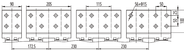
水平接线及相间距
