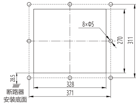
RDW7-4000 ~ 6300固定式断路器面板开孔尺寸
