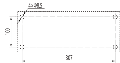
安装尺寸示意图
