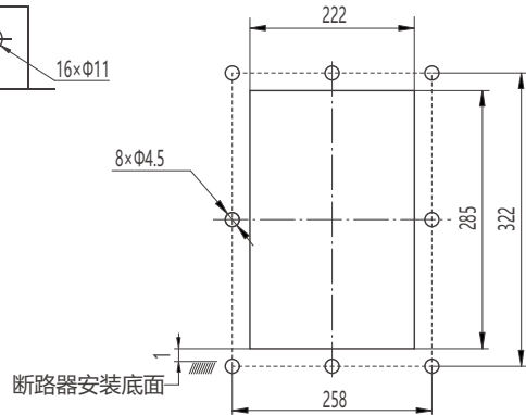
RDW7-1600S固定式断路器面板开孔尺寸
