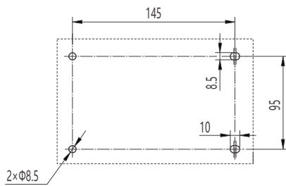
安装尺寸示意图
