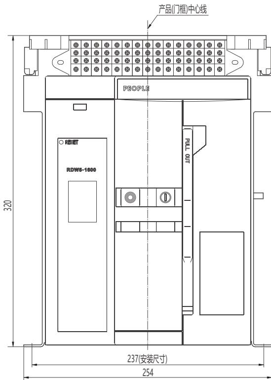
中心线及外形尺寸
