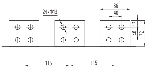
4000水平接线及相间距(2500/3200可选)
