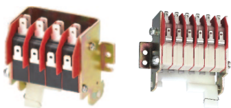
RDW7-1600(S)辅助开关
