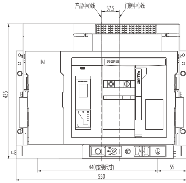
中心线及外形尺寸
