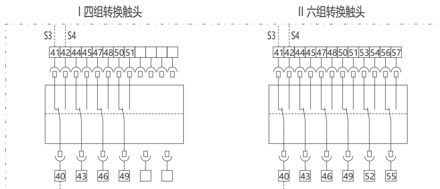
RDW7-1600H型二次回路接线图
