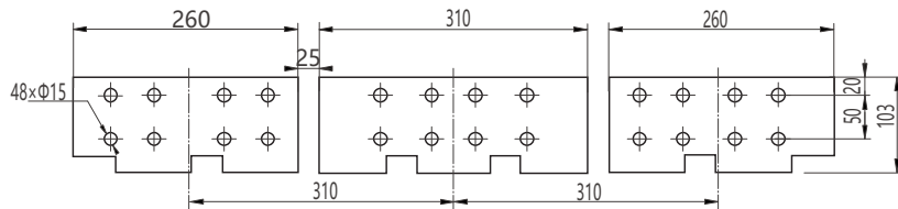
三极极水平接线及相间距
