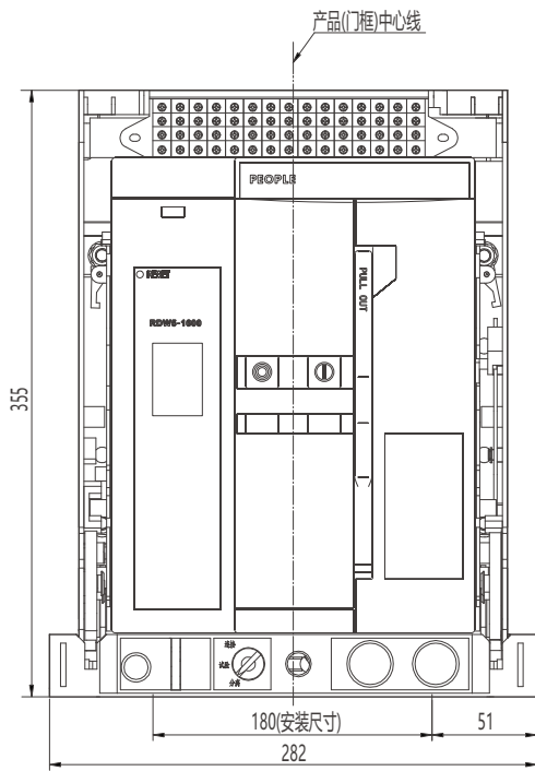
中心线及外形尺寸
