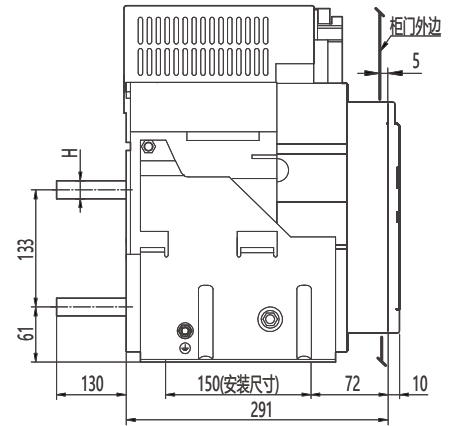
水平接线及外形尺寸
