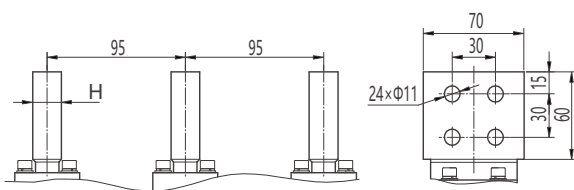
垂直接线及相间距
