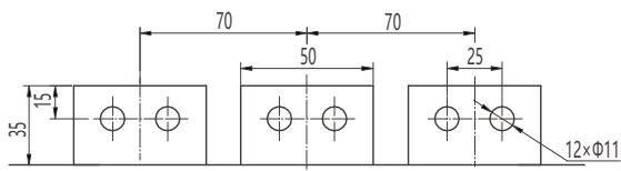
中心线及外形尺寸
