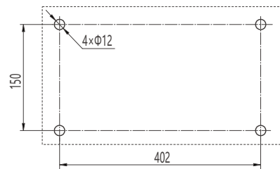
安装尺寸示意图
