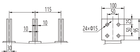
垂直接线及相间距
