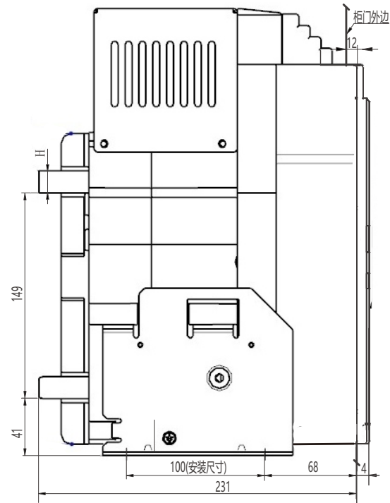
水平接线及外形尺寸
