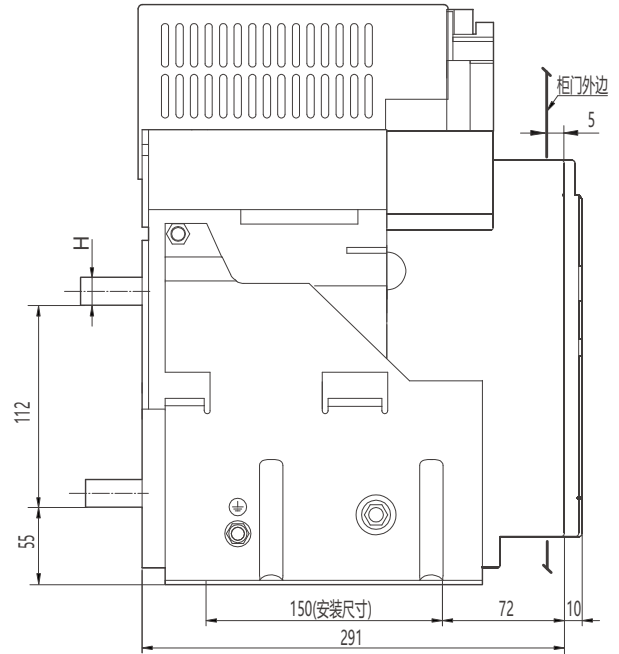
水平接线及外形尺寸
