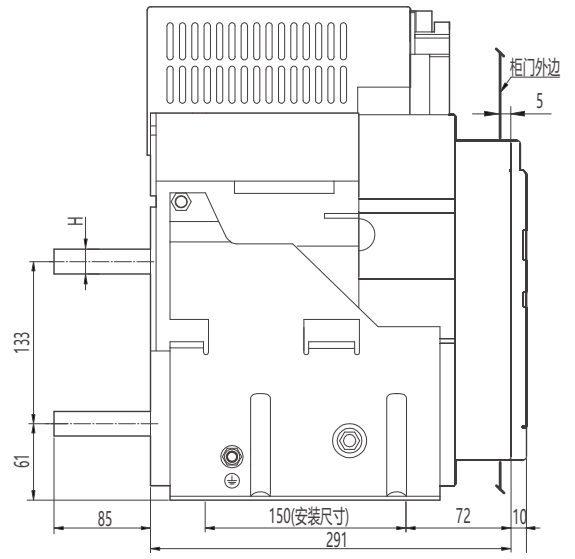
水平接线及外形尺寸
