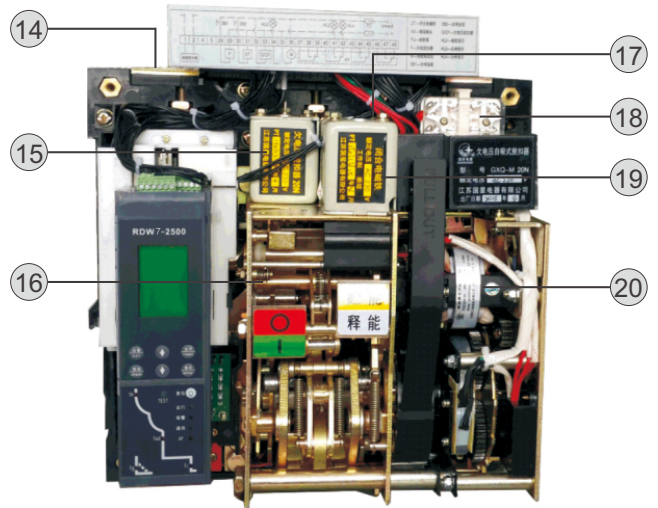
断路器本体
