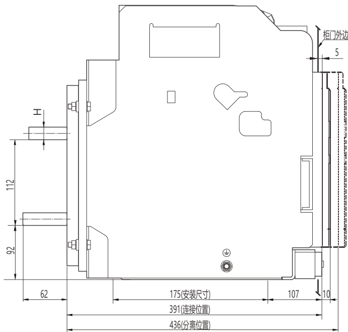
水平接线及外形尺寸
