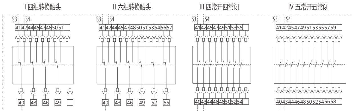
RDW7-2500 ~ 6300H型二次回路接线图
