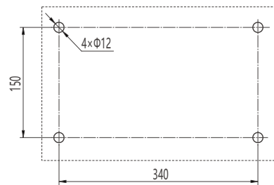
安装尺寸示意图
