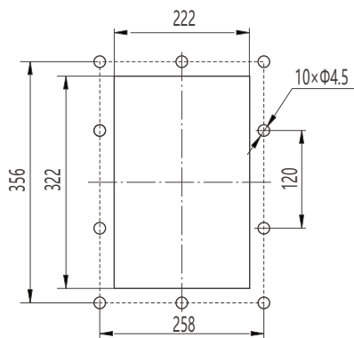
RDW7-1600抽屉式断路器面板开孔尺寸
