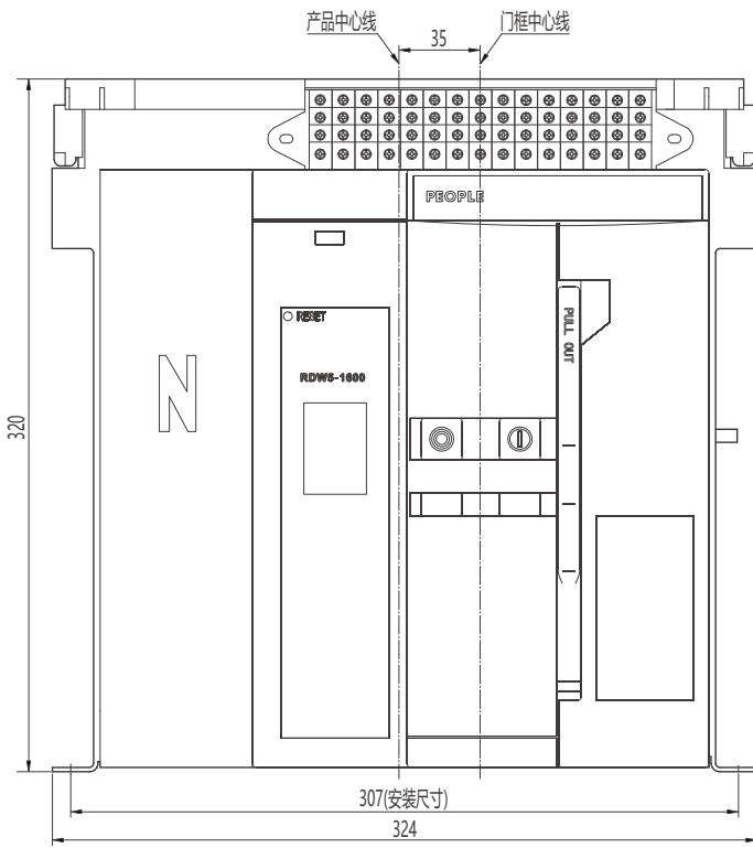
中心线及外形尺寸
