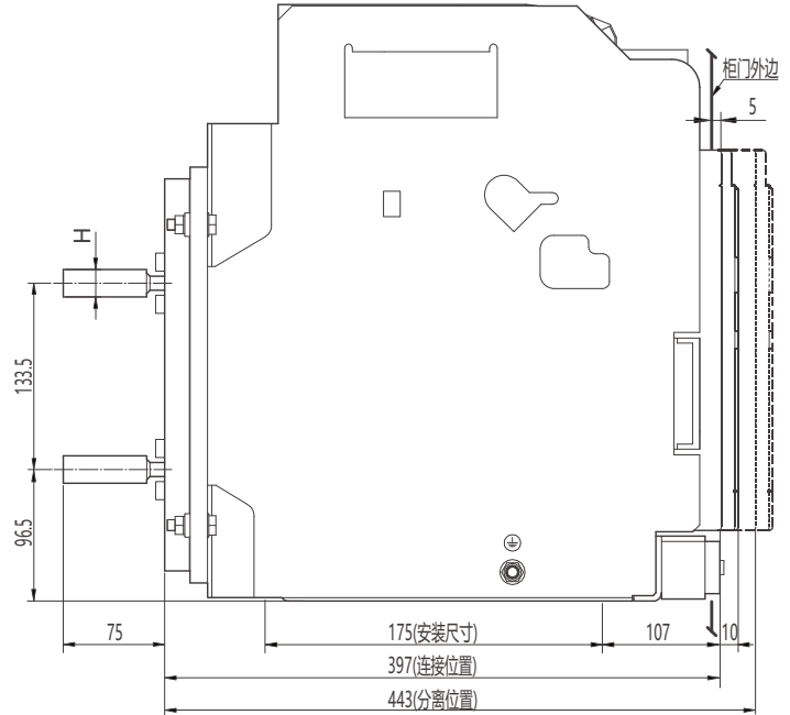
水平接线及外形尺寸
