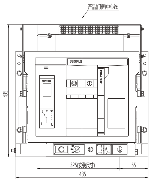
中心线及外形尺寸
