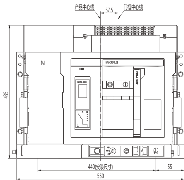
中心线及外形尺寸
