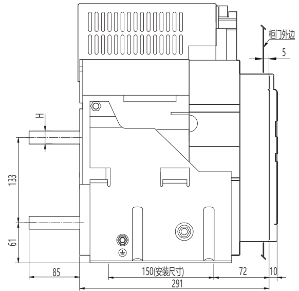
水平接线及外形尺寸
