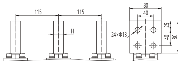
垂直接线及相间距
