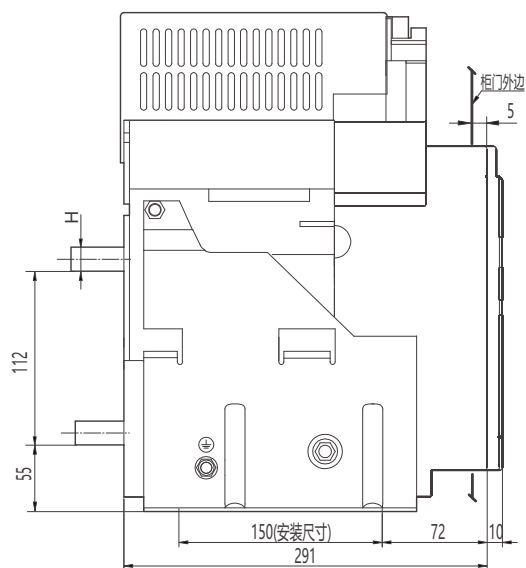
水平接线及外形尺寸
