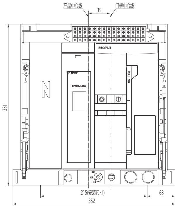
中心线及外形尺寸
