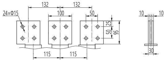
水平接线及相间距
