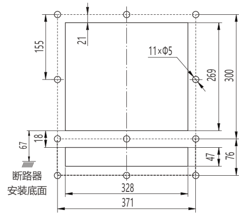
RDW7-4000~6300抽屉式断路器面板开孔尺寸
