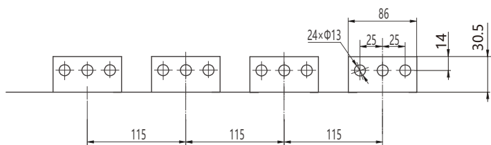
2500、3200水平接线及相间距
