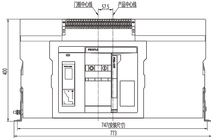
中心线及外形尺寸
