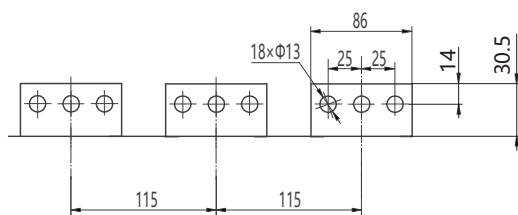
2500、3200水平接线及相间距
