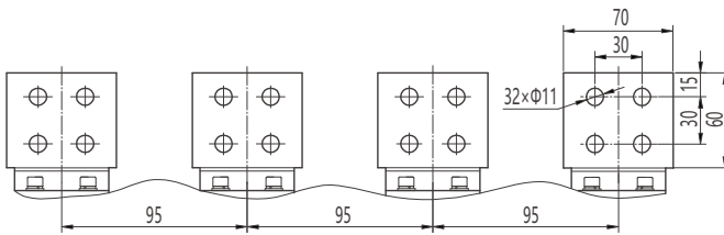
水平接线及相间距
