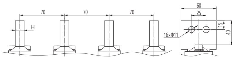
垂直接线及相间距
